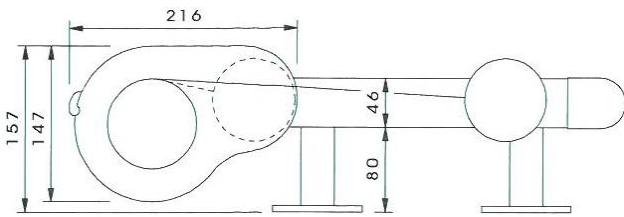
Seitenansicht
