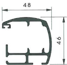
Führungsschiene
