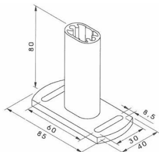
Standard-Montagekonsole
