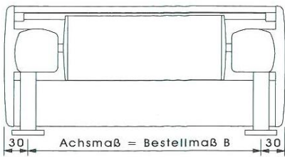
Vorderansicht einteilig
