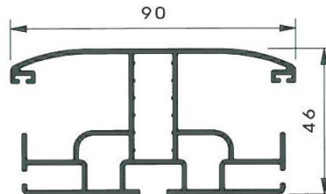
Mittelführungsschiene
